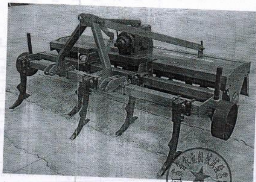
1SZL-230 深松整地联合作业机 (参与产品研发人员:王万军 汪春辉 蔡发全 张国和)
